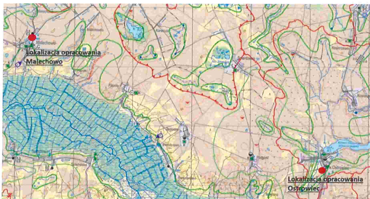
Ryc. 3. Lokalizacja opracowania na tle mapy hydrograficznej (źródło: http://geoserwis.gdos.gov.pl/mapy/ ).
